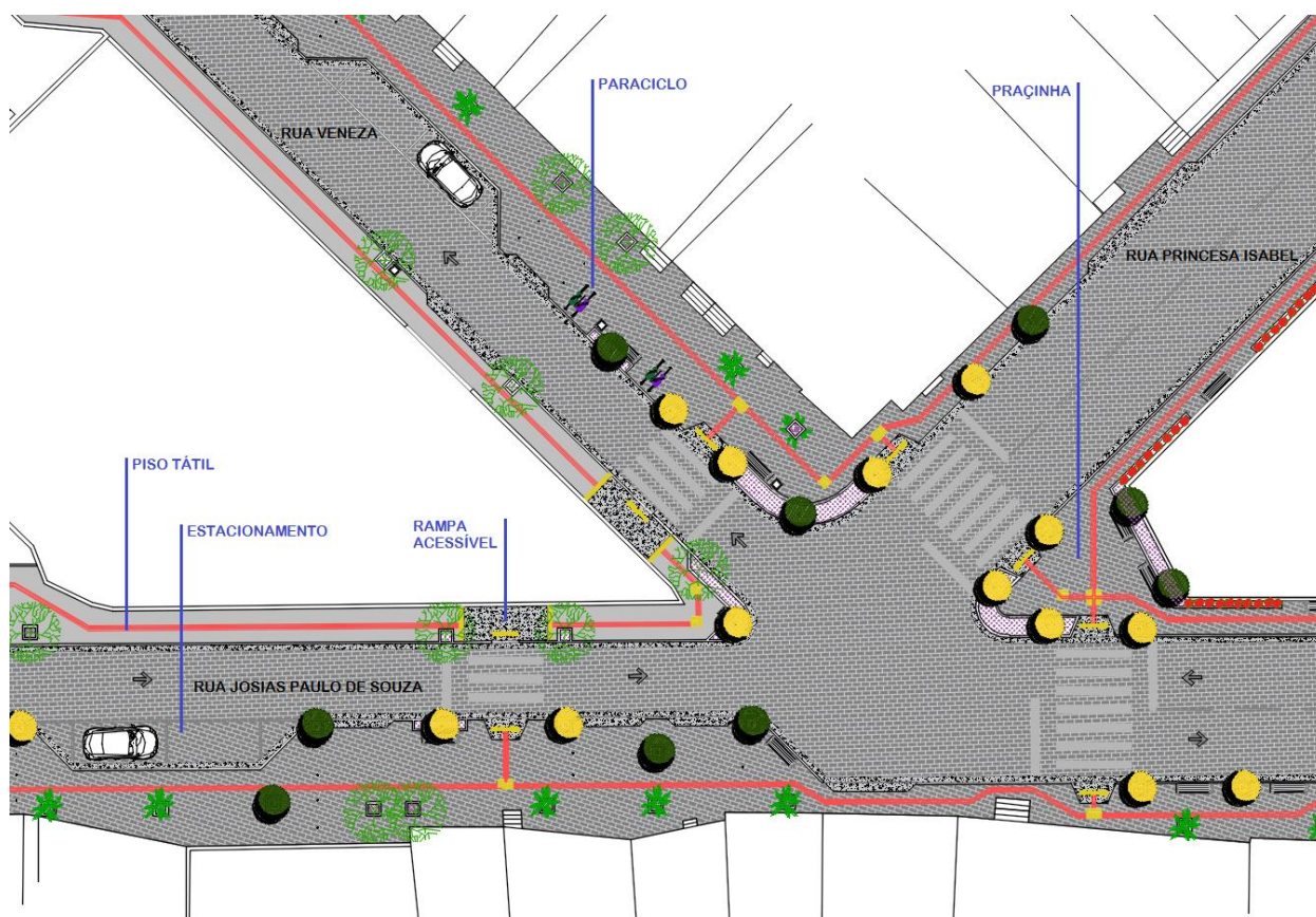
Imagem 14 – Imagem trecho da intervenção no Vicente Pinzón: planta-baixa. Fonte: COPROJ-SEINF.
