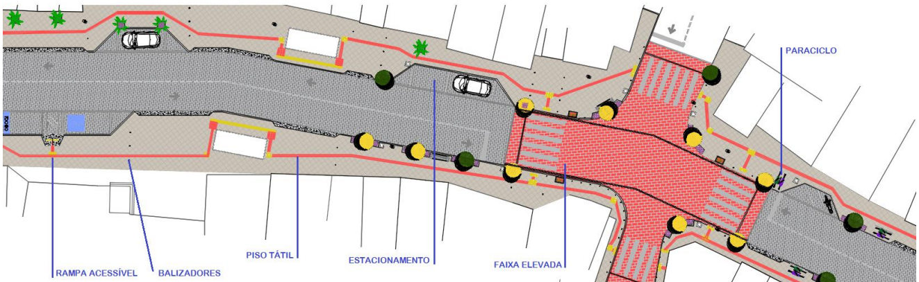
Imagem 11 – Trecho do projeto no Serviluz: planta-baixa. Fonte: COPROJ-SEINF.
